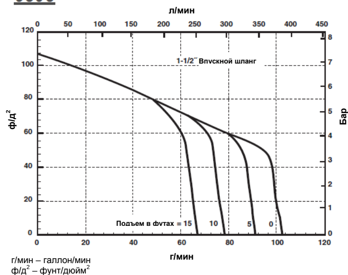
Производительность 9303C-HM1C-SP при 13 г/мин
